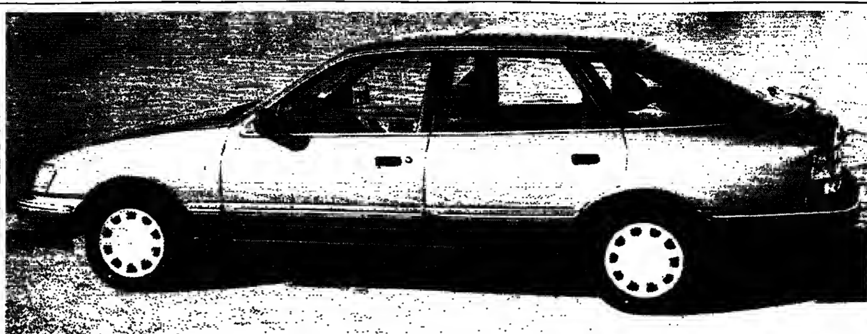
Gelungene Synthese aus Aerodynamik, Funktionalität und Optik. Mit einem Luftwiderstandsbeiwert von 0,33 ergibt sich für den Scorpio eine Verringerung des Luftwiderstands um rund 30 Prozent im Vergleich zum Vorgänger.
